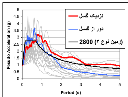
شکل ۴- مقایسه طیف میانگین به علاوه انحراف معیار نزدیک و دور از گسل با طیف استاندارد ۲۸۰۰ و برایش ۳. (۵٪)
