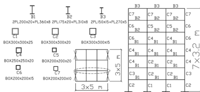
شکل ۲- شکل هندسی و مشخصات مقاطع مدل سازه ای
