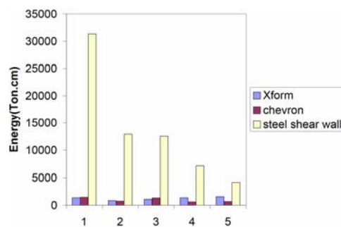
شکل ۸- میزان استهلاک انرژی (۱:قابهای ۱، ۱۶، ۱۲- ۲:قابهای ۲، ۷، ۱۲- ۳:قابهای ۳، ۸، ۱۳- ۴:قابهای ۴، ۹، ۱۴- ۵:قابهای ۵، ۱۰، ۱۵)
