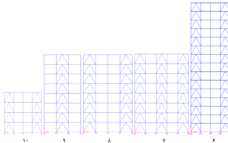
شکل ۵- قابهای دارای سیستم دوگانه قاب خمشی متوسط و بادبند شورون
