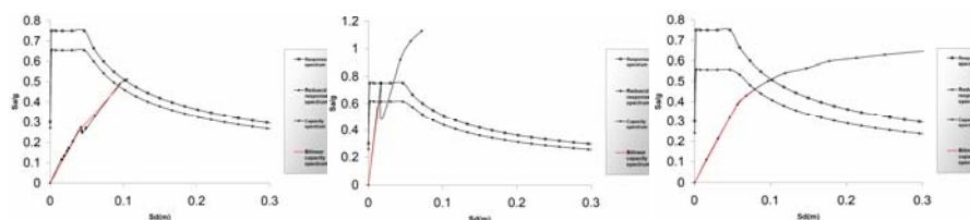
شکل ۷- نقطه عملکرد قاب ۱۵ (سمت راست)، قاب ۱۰ (وسط)، قاب ۵ (سمت چپ)
