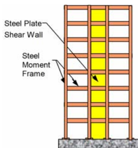
شکل ۲- دیوار برشی فولادی و قاب خمشی محیطی
