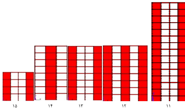
شکل ۶- قابهای دارای سیستم دوگانه قاب خمشی متوسط و دیوار برشی فولادی نازک
