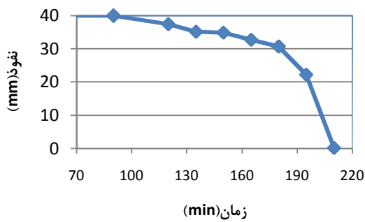
شکل ۱۰- نمودار آزمایش زمان گیرش برای سیمان ۸۵٪
