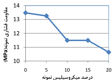
شکل ۱۷- نمودار مقاومت فشاری بر حسب مقدار میکروسیلیس
