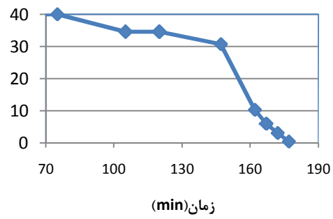
شکل ۹- نمودار آزمایش زمان گیرش برای سیمان ۹۰٪
