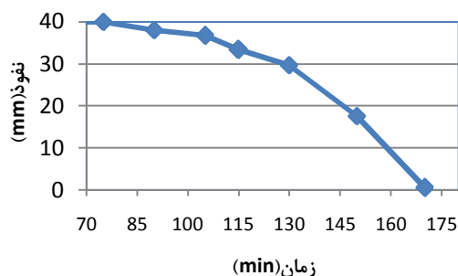
شکل ۸- نمودار آزمایش زمان گیرش برای سیمان ۹۵٪
