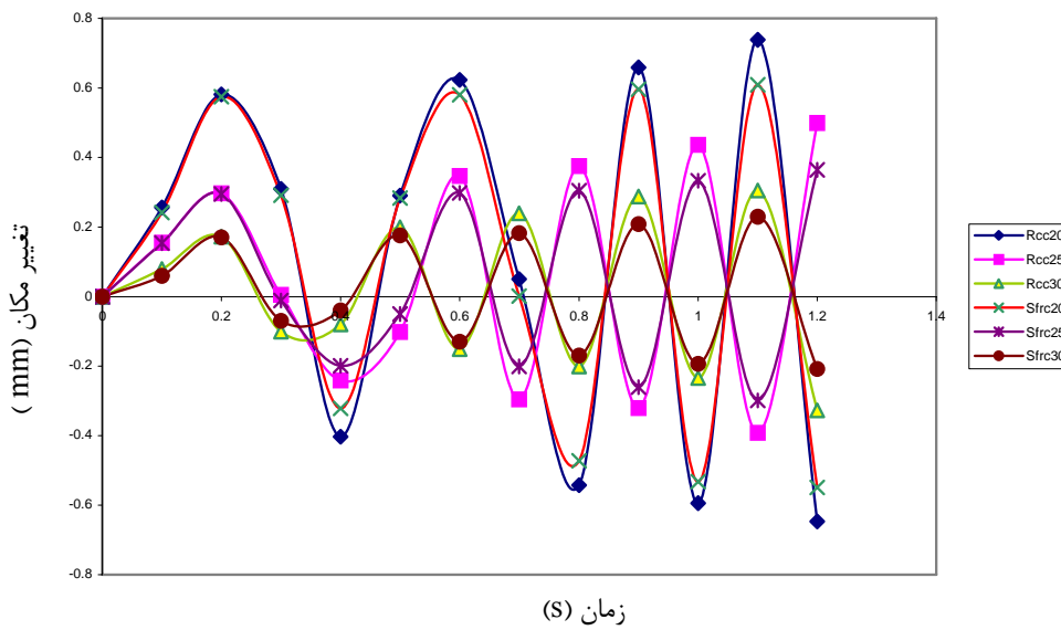
شکل ۳ - مقایسه تغییر مکان صفحات RCC و SFRC با ضخامتهای ۲۰، ۲۵ و ۳۰ میلیمتر با تکیه گاه گیردار در ۴ جهت
