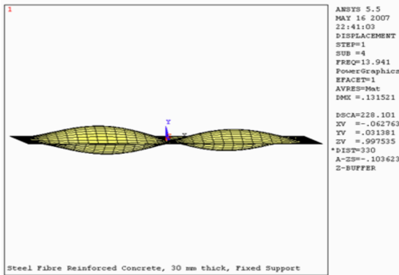
شکل ۵ - مد شکل شماره ۴ صفحه SFRC با ضخامت ۳۰ میلیمتر و گیردار
