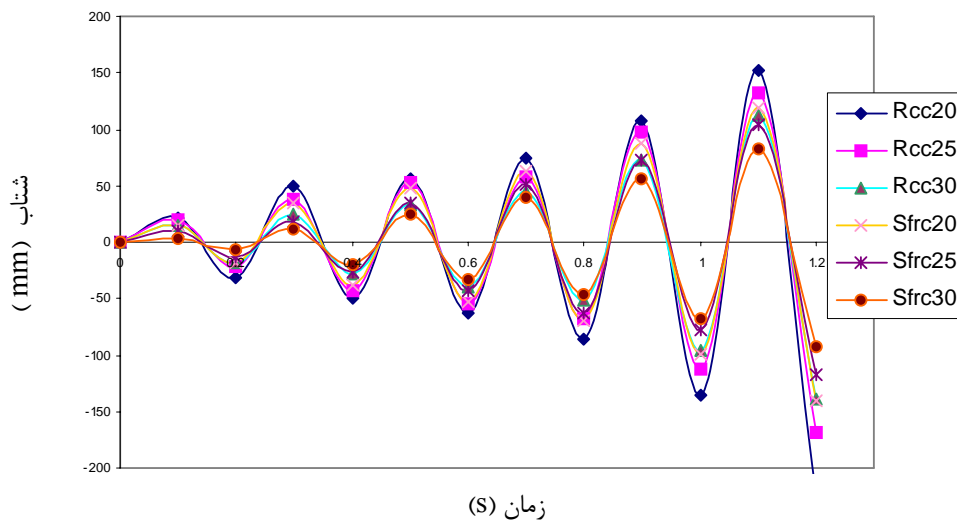
شکل ۴ - مقایسه شتاب صفحات RCC و SFRC با ضخامتهای ۲۰، ۲۵ و ۳۰ میلیمتر با تکیه گاه گیردار در ۴ جهت
