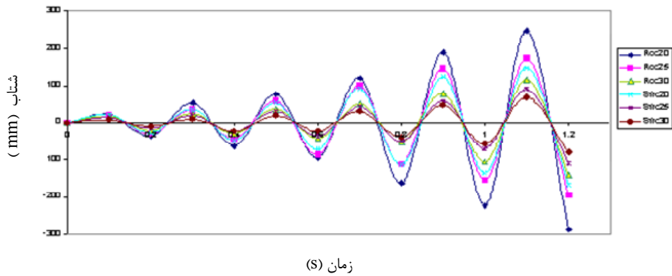
شکل ۲ - مقایسه شتاب صفحات RCC و SFRC با ضخامتهای ۲۰، ۲۵ و ۳۰ میلیمتر با تکیه گاه ساده در ۴ جهت
