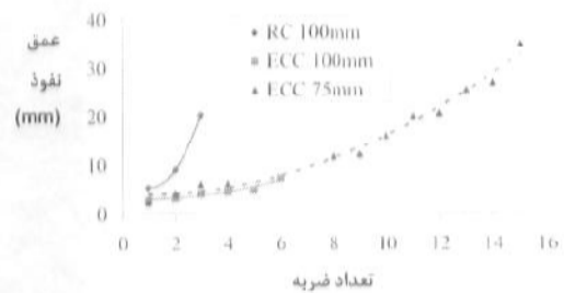
شکل ۸- عمق نفوذ بر حسب تعداد ضربه ها
