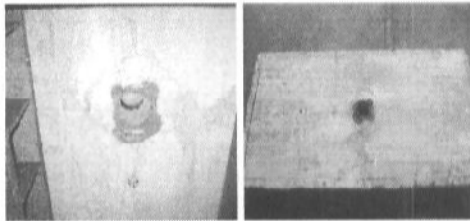
شکل ۷- وجه پشتی ECC75 پس از هفدهمین ضربه
