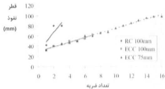
شکل ۹- قطر نفوذ بر حسب تعداد ضربه ها
