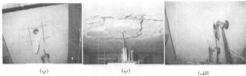
شکل ۴- آسیب وارده بر وجه پشتی پانل RC100: (الف) پس از اولین ضربه، (ب) پس از دومین ضربه (قلوه‌کن شدن زیاد)، (پ) پس از سومین ضربه (عبور کامل با ایجاد مخروط برشی بزرگ- الگوی ترک خوردگی)
