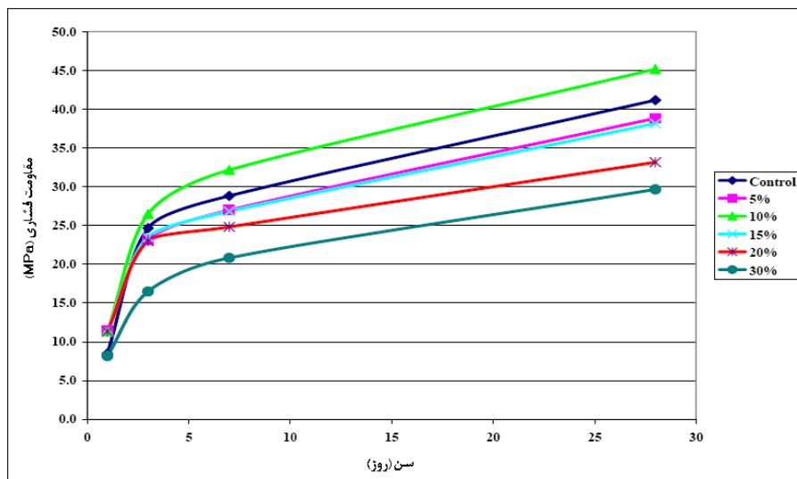
شکل ۳- مقایسه مقاومت فشاری نمونه های بتنی با جایگزینی مقادیر متقاومت متاکائولین
