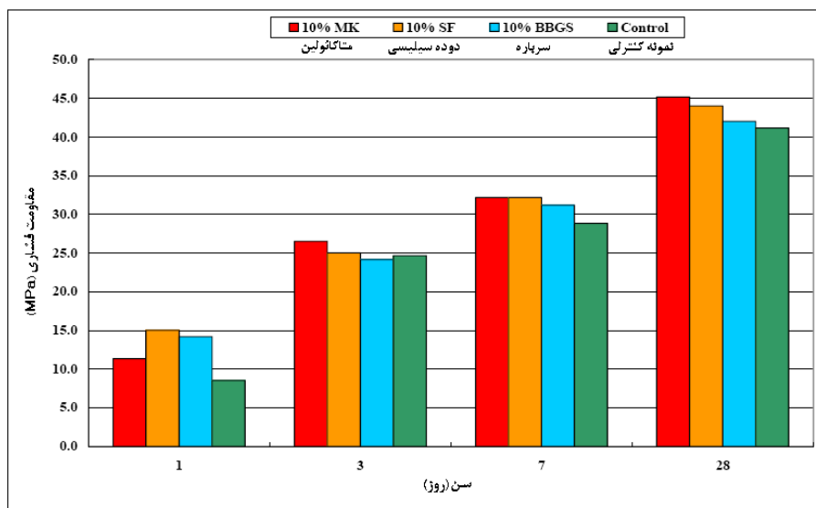
شکل ۵- مقایسه مقاومت فشاری نمونه ای با جایگزینی مقادیر یکسان متاکائولین (MK)، دوده سیلیسی (SF) و سربراره (BBS)
