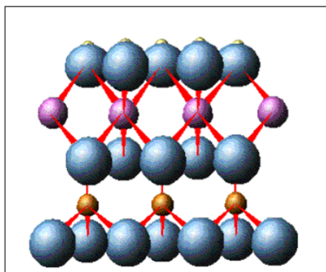
شکل ۲- ساختار کائولینیت
